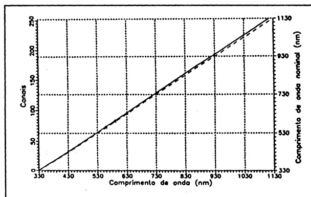
Fig. 3 Calibração espectral do espectrorradiômetro SE 590 S/N 1445.
