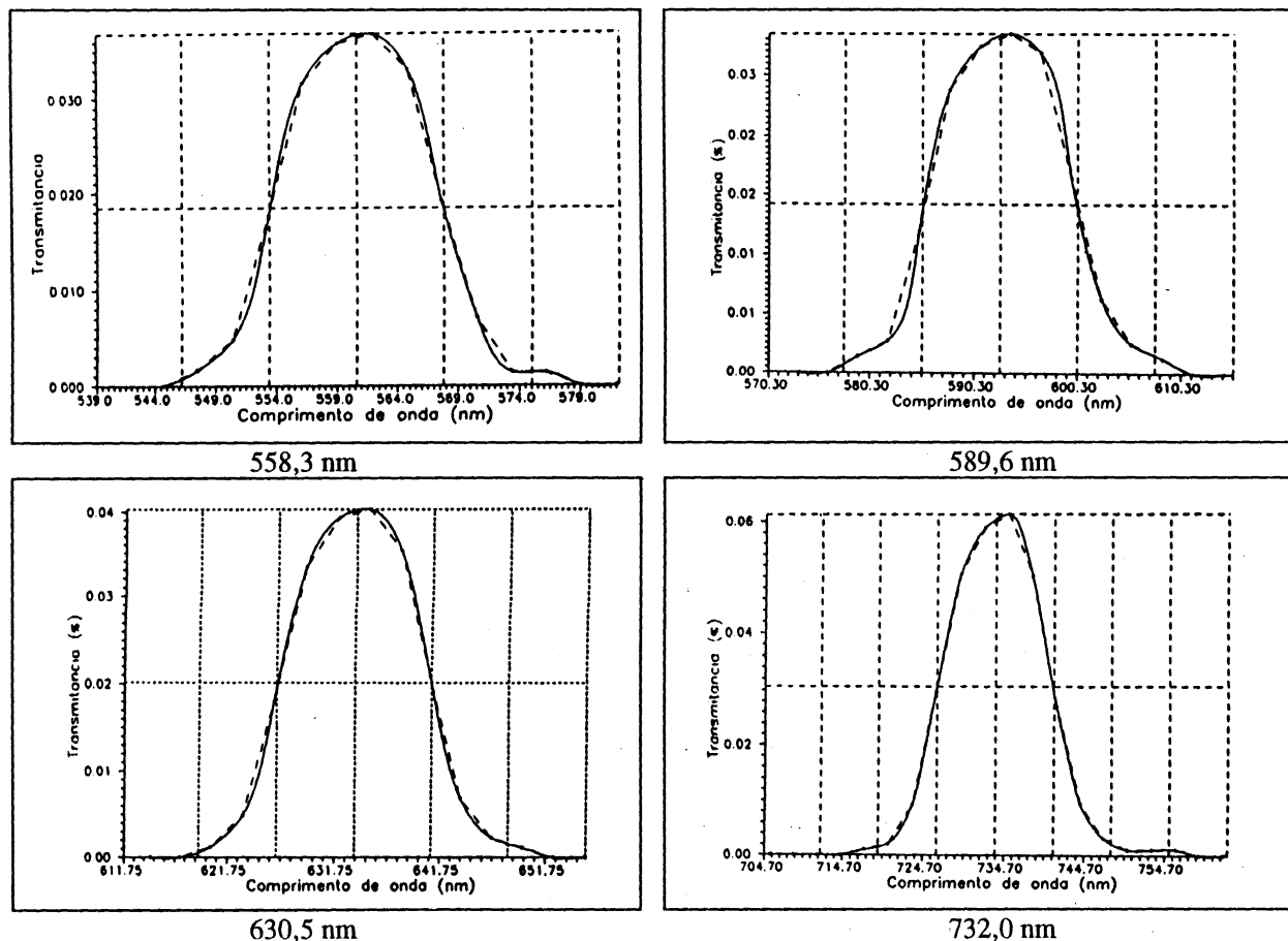
Fig. 2. Gráfico representativo da transmitância obtida no espectrorradiômetro SE-590 para o filtros interferométricos 558,3 nm, 589,6 nm, 630,5 nm, 732,0 nm.
